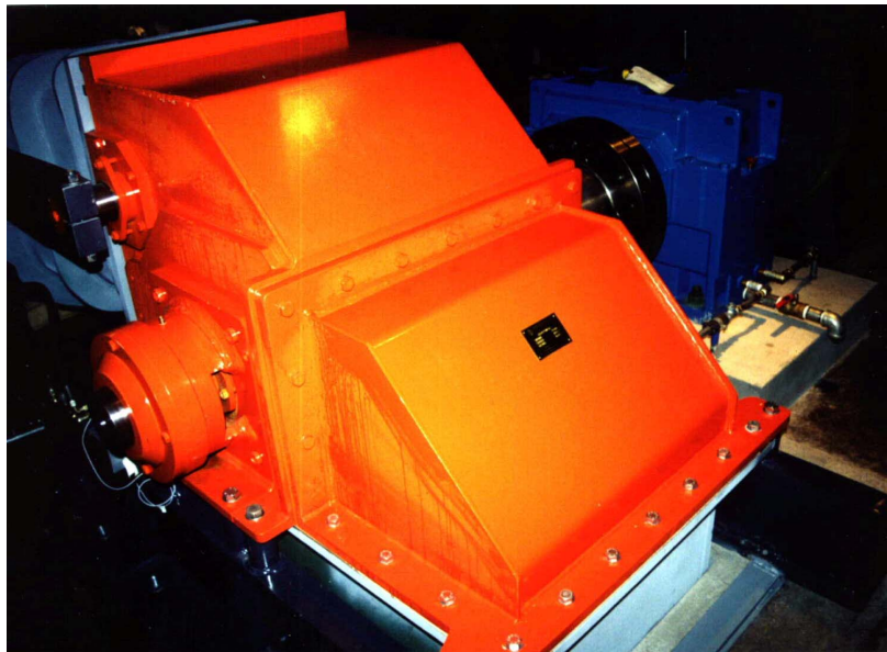
Abb. 5: OSSBERGER Durchström-Turbine Type G6.039/12g
