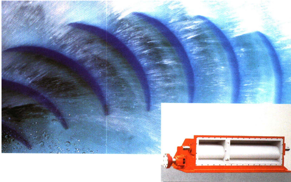
Abb. 6: Patentierte OSSBERGER-Durchström-Turbine - Blick auf Einlaufseite, Leitschaufeln aufgeteilt im Verhältnis 1:2 Antriebswelle mit Kupplung, links halb sichtbar
