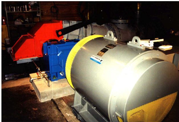
Abb. 3: Nach Fertigstellung, vorn der 450 kW-Induktionsgenerator
