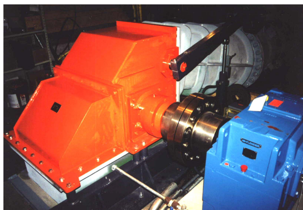
Abb. 4: Die neue OSSBERGER Durchström-Turbine mit FLENDER- Getriebe und flexibler Kupplung; eingebaut an der Anlage Maroon Creek Hydro, stellt eine zuverlässige Kombination mit hoher Leistung dar.
